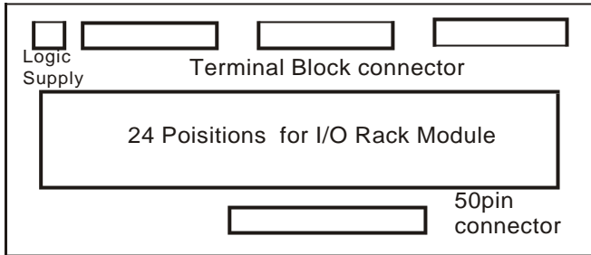
DIN-24G Outline
